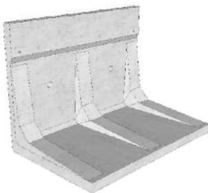
■控え壁形状 (H1000～H3500)
